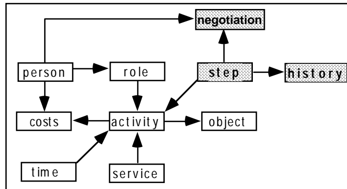
Abbildung 2: Erweitertes FUNSOFT-Metamodell nach [DGS95]
