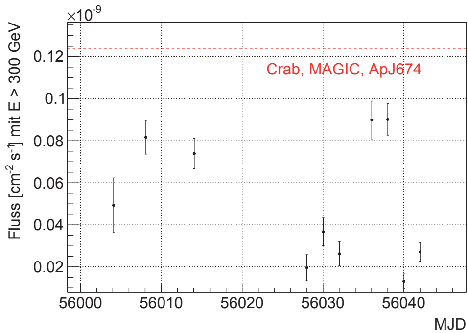
Abbildung 4.8: Lichtkurve von Mrk 421 im Zeitraum vom 18.3.2012 bis zum 25.4.2012. Der Fluss von Mrk 421 liegt im Durchschnitt bei 41% des Flusses von Crab, den die rote Linie darstellt.
