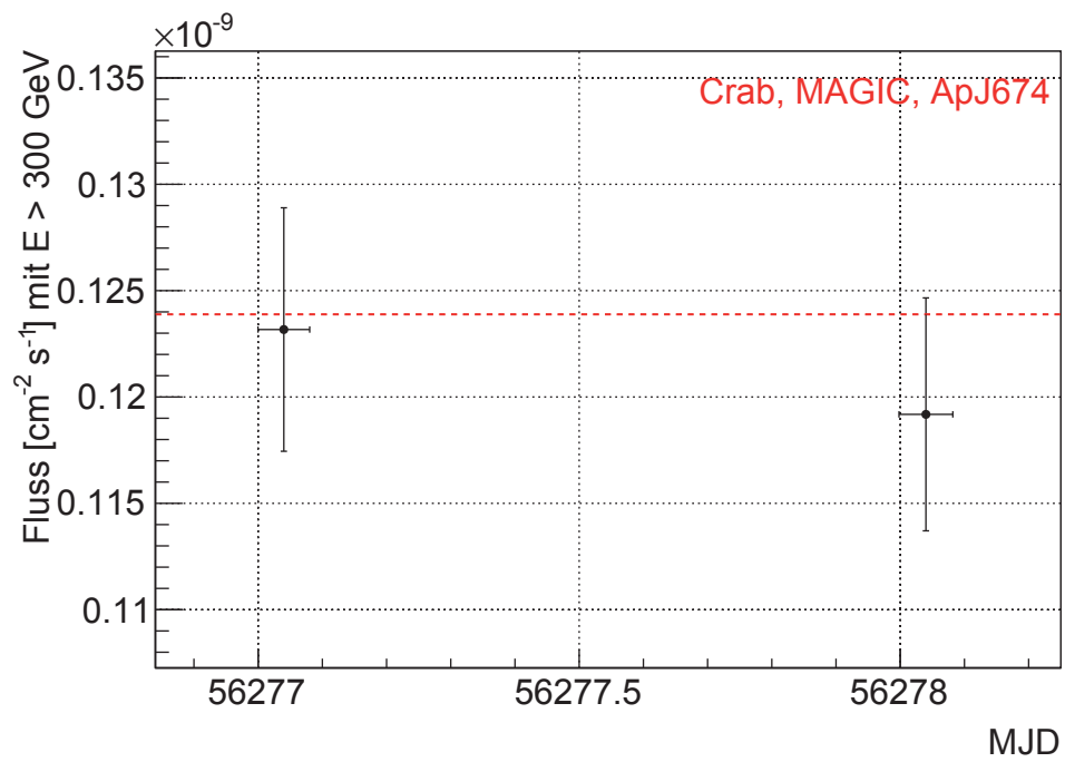
Abbildung 4.15: Lichtkurve von Crab im Zeitraum vom 15.12.2012 bis zum 23.12.2012 mit dem mittleren Crab-Fluss (nach [7]).
