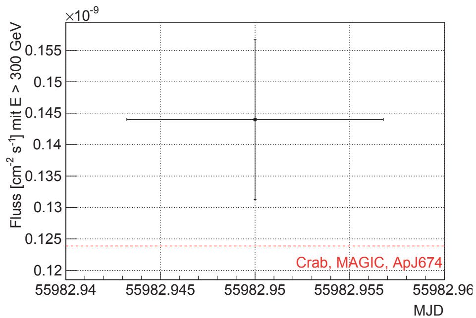
Abbildung 4.12: Lichtkurve von Crab im Zeitraum vom 25.2.2012 bis zum 29.2.2012 mit dem mittleren Crab-Fluss (nach [7]).
