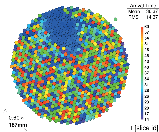
Abbildung 3.5: Darstellung der Ankunftszeiten eines Schauers in der Kamera. Dargestellt sind die Ankunftszeiten in time slices. Die Pixel, die zum Schauer gehören, weisen ähnliche Ankunftszeiten auf, während die übrigen Pixel zufällig verteilte Werte für die Ankunftszeit zeigen.
