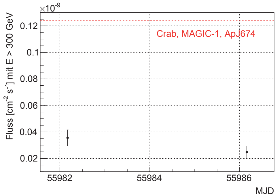
Abbildung 4.13: Lichtkurve von Mrk 421 im Zeitraum vom 25.2.2012 bis zum 29.2.2012. Der Fluss von Mrk 421 liegt im Durchschnitt bei 24% des Flusses von Crab, den die rote Linie darstellt.
