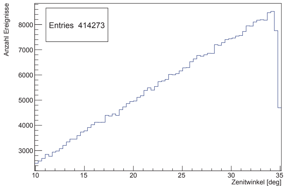
Abbildung 4.6: Zenitverteilung des Trainingssets der MC.
