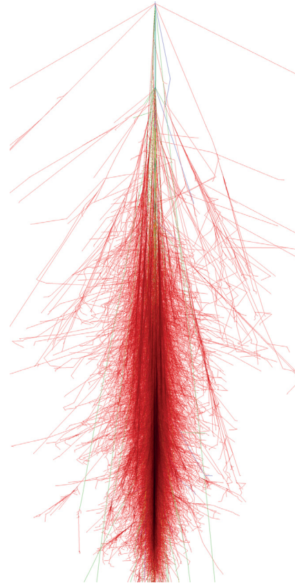
(b) Simulation eines Schauers mit einem 1 TeV-Proton als Primärteilchen.
