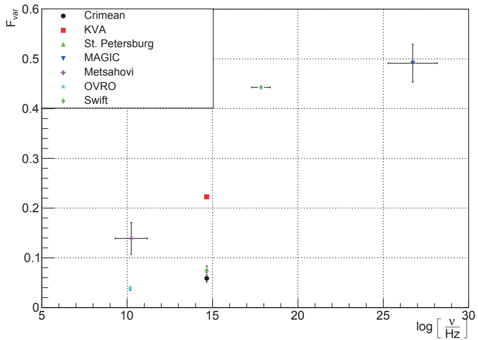
Abbildung 5.2: Darstellung der Variabilitäten in den verschiedenen Wellenlängen. Es ist zu erkennen, dass mit steigender Frequenz die Variabilität zunimmt. Die Variabilität der Röntgen- und der Gammastrahlung ist auf einem ähnlichen Niveau.
