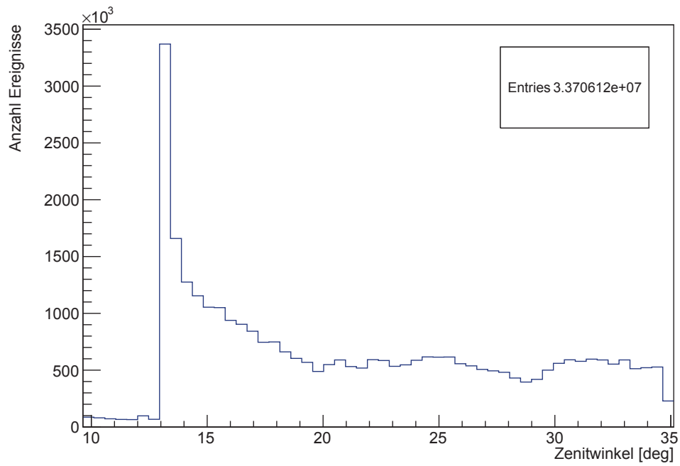
Abbildung 4.5: Zenitverteilung der Background-Daten zwischen dem 18.3.2012 und dem 27.4.2012.
