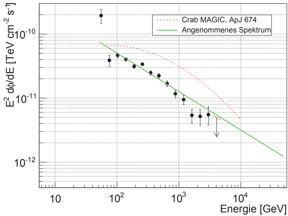
Abbildung 4.9: Spektrale Energieverteilung von Mrk 421. Zum Vergleich ist die spektrale Energieverteilung von Crab in rot eingezeichnet.
