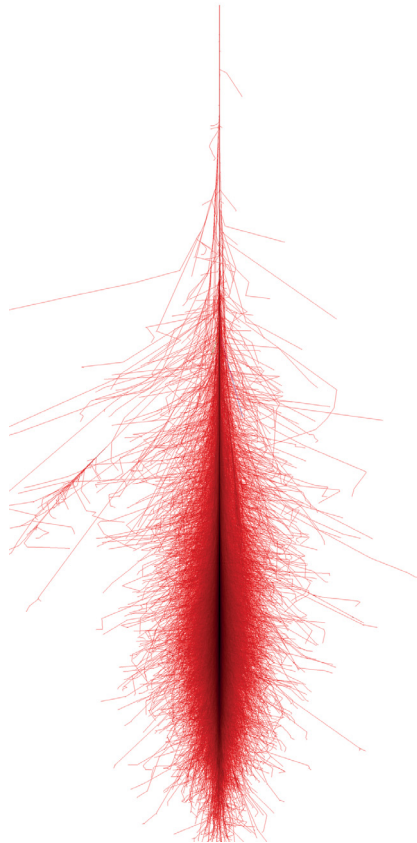
(a) Simulation eines Schauers mit einem 1 TeV-Photon als Primärteilchen.
