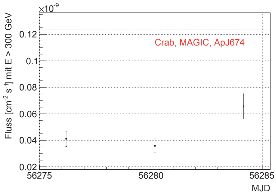
Abbildung 4.16: Lichtkurve von Mrk 421 im Zeitraum vom 15.12.2012 bis zum 23.12.2012. Der Fluss von Mrk 421 liegt im Durchschnitt bei 38% des Flusses von Crab, den die rote Linie darstellt.
