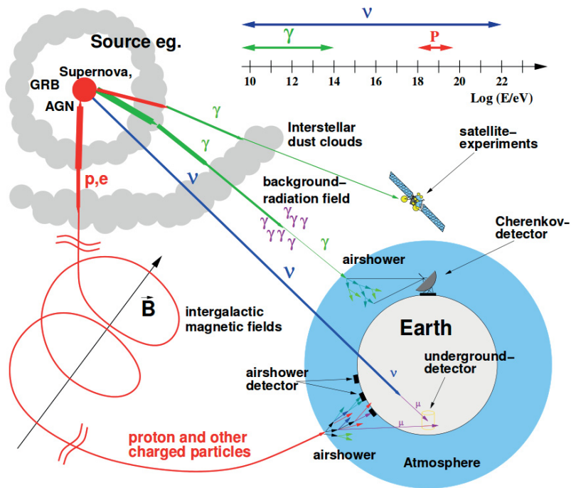
Abbildung 2.1: Schematische Darstellung der Wechselwirkungen der Botenteilchen auf dem Weg von der Quelle zum Beobachter sowie ihrer Detektion. Auf ihrem Weg unterliegen die unterschiedlichen Botenteilchen unterschiedlichen Wechselwirkungen. Geladene Teilchen wechselwirken mit Staubwolken und werden von Magnetfeldern abgelenkt, Neutrinos und hochenergetische Photonen behalten ihre Richtungsinformation bei. Photonen wechselwirken ebenfalls mit Staubwolken oder mit niederenergetischen Hintergrundphotonen und werden dann abhängig von ihrer Energie mit unterschiedlichen Detektoren gemessen. Das Bild entstammt [24].
