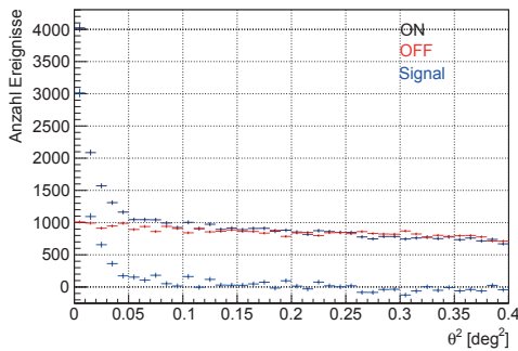
(a) \theta^2 -Plot für Crab für alle Wobble-Positionen
