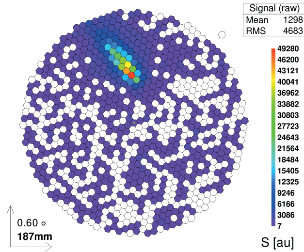
Abbildung 3.3: Darstellung eines simulierten Schauers mit einer Primärteilchenenergie von 3,0 TeV in der Kamera. Die Farbskala zeigt den simulierten Photoneninhalt in den einzelnen Pixeln in beliebigen Einheiten.
