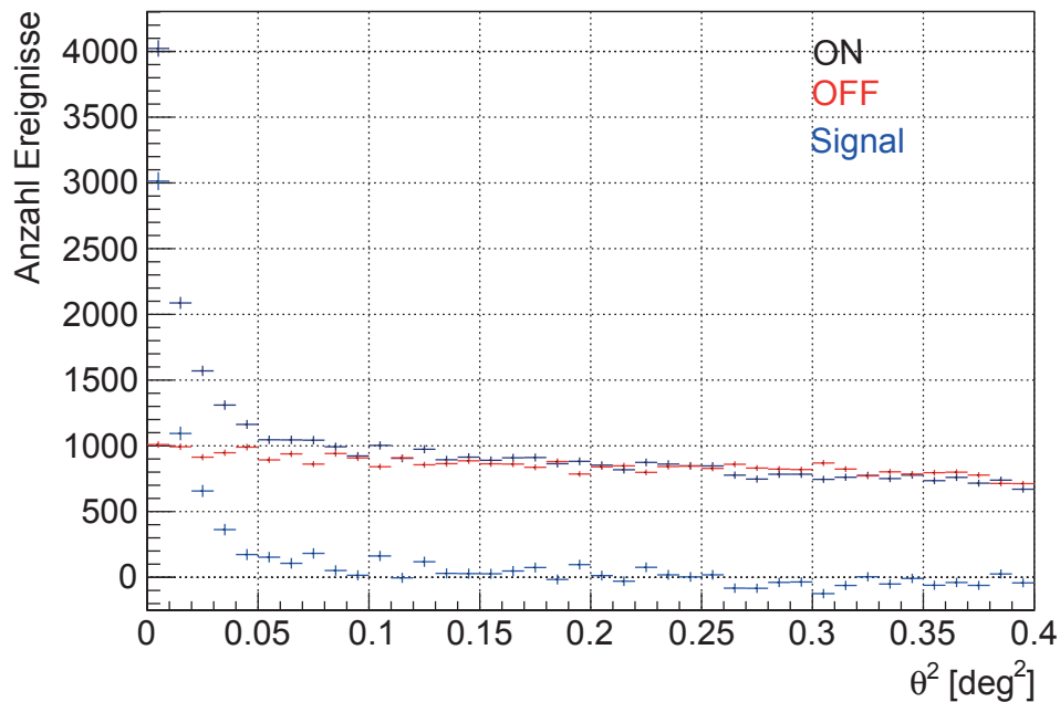
Abbildung 4.2: \theta^2 -Verteilung von Crab-Daten aus dem Datensatz 2. Es ist zu sehen, dass die On- (schwarz) und die Off-Daten (rot) für \theta^2 > 0,1 miteinander übereinstimmen. Des Weiteren werden die Signal-Daten in blau dargestellt, die sich aus den On-Daten nach Subtraktion der Off-Daten ergeben. Ereignisse aus der Quelle befinden sich wie erwartet bei \theta^2 \approx 0 .
