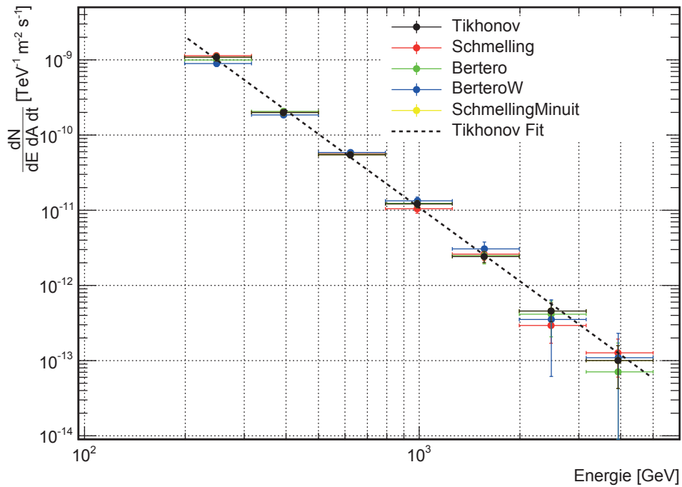
Abbildung 4.19: Spektrum von Mrk 421 im Zeitraum vom 23.05.2012 bis zum 19.06.2012 mit allen wählbaren Regularisierungsmethoden. Die gestrichelte Linie stellt das gefittete Spektrum dar, welches mit Hilfe der Tikhonov-Regularisierung berechnet wurde.
