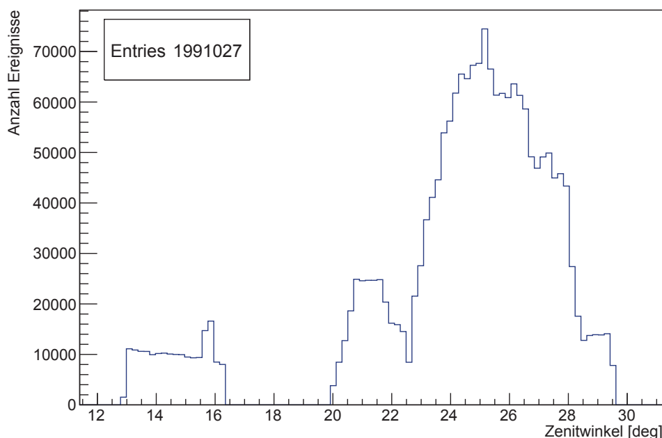
Abbildung 4.4: Zenitverteilung der genommenen Mrk 421-Daten zwischen dem 18.3.2012 und dem 27.4.2012.
