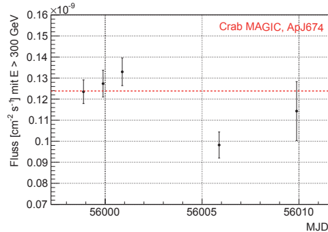
(d) Lichtkurve von Crab mit mittlerem Fluss von Crab, berechnet nach [7].
