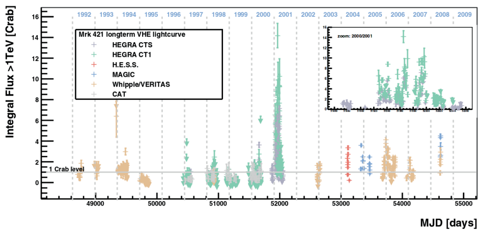
Abbildung 2.5: Die Abbildung zeigt eine Lichtkurve von Mrk 421, die zwischen 1992 und 2009 aufgenommen wurde. Die Variabilität dieser Quelle ist deutlich zu erkennen, wobei 2001 die größte Aktivität herrschte.[63]
