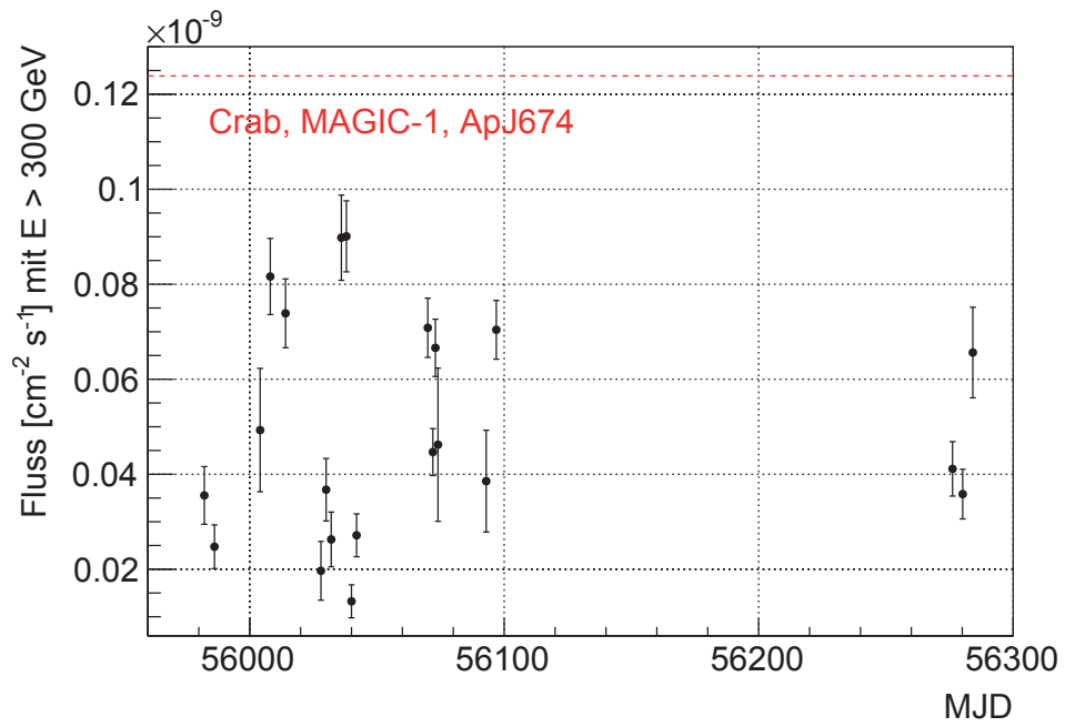
Abbildung 4.20: Zusammenfassende Lichtkurve der Mrk 421-Daten. Es sind alle vorher berechneten Lichtkurven-Daten in einem Diagramm dargestellt. Es ist zu sehen, dass der Fluss von Mrk 421 im gesamten Jahr 2012 unterhalb des mittleren Flusses von Crab liegt, allerdings durchaus zeitliche Variabilitäten aufweist.
