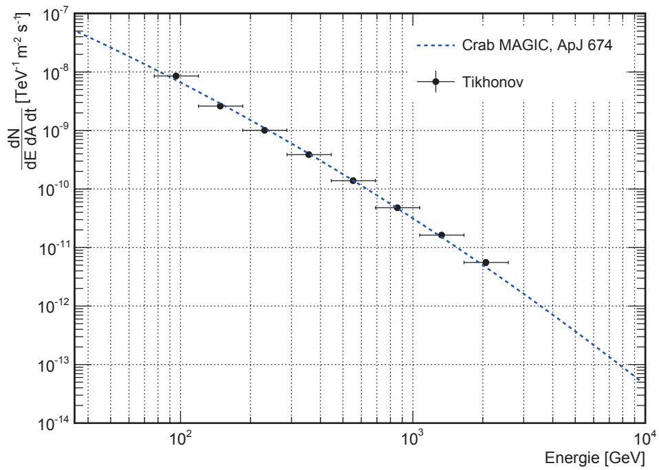
Abbildung 4.10: Entfaltetes Crab-Spektrum im Zeitraum vom 18.3.2012 bis zum 25.4.2012 mit einem Literaturvergleich (siehe [7]).
