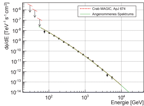
(b) Differenzielles Energiespektrum
