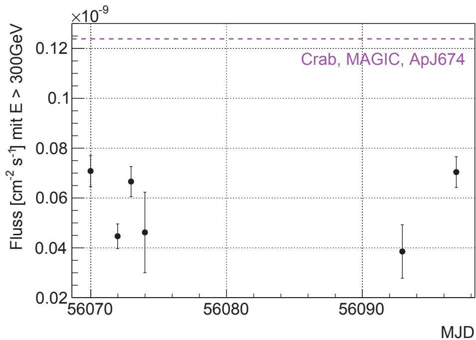
Abbildung 4.18: Lichtkurve von Mrk 421 im Zeitraum vom 23.05.2012 bis zum 19.06.2012. Der Fluss von Mrk 421 liegt im Durchschnitt bei 45% des Flusses von Crab, den die rosa Linie darstellt.
