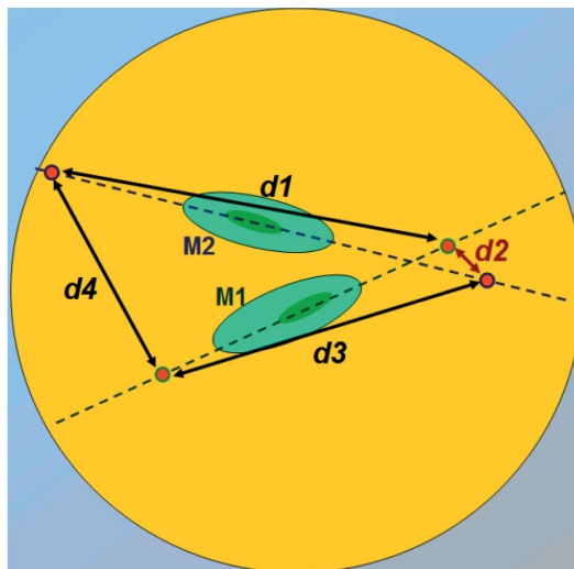
Abbildung 4.1: Schema zur Rekonstruktion des Stereo-Parameters Disp . Dargestellt sind die aufgenommenen Schauer beider Kameras, projiziert auf eine Kameraebene. Die roten Punkte stellen die möglichen Quellpositionen des Schauers in der Kamera von MAGIC-I (im Bild: M1) und MAGIC-II (im Bild: M2) dar. Die Abstände zwischen den rekonstruierten Quellpositionen der beiden Teleskope werden durch d_i dargestellt. Der kleinste Wert für d_i beschreibt hier den Abstand zwischen den beiden wahrscheinlicheren Disp -Werten. Aus den Abständen dieser Punkte zueinander kann entschieden werden, welche Herkunftsrichtung für den Schauer am wahrscheinlichsten ist.[44]
