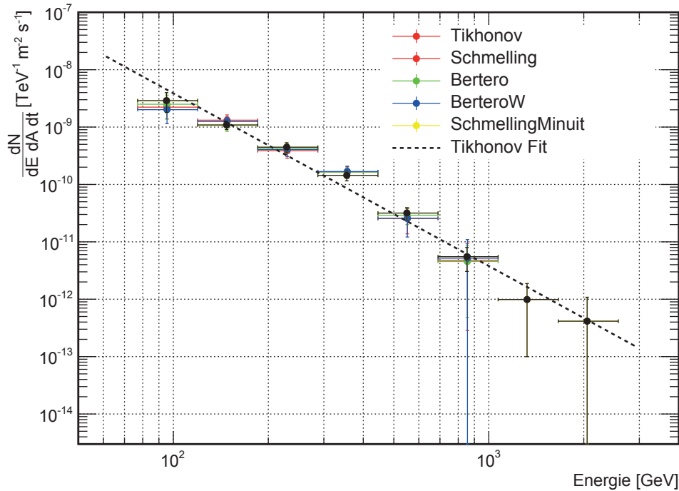
Abbildung 4.14: Entfaltetes Spektrum von Mrk 421 im Zeitraum vom 25.2.2012 bis zum 29.2.2012 mit allen wählbaren Regularisierungsmethoden. Die gestrichelte Linie stellt das gefittete Spektrum dar, welches mit Hilfe der Tikhonov-Regularisierung berechnet wurde.
