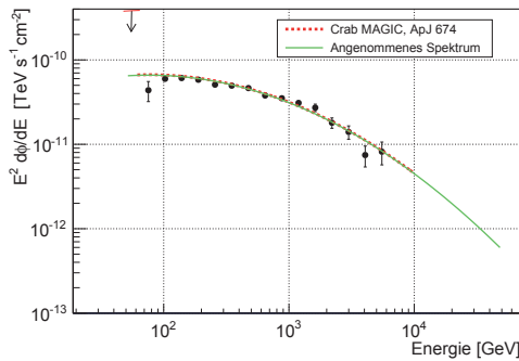
(c) Spektrale Energieverteilung
