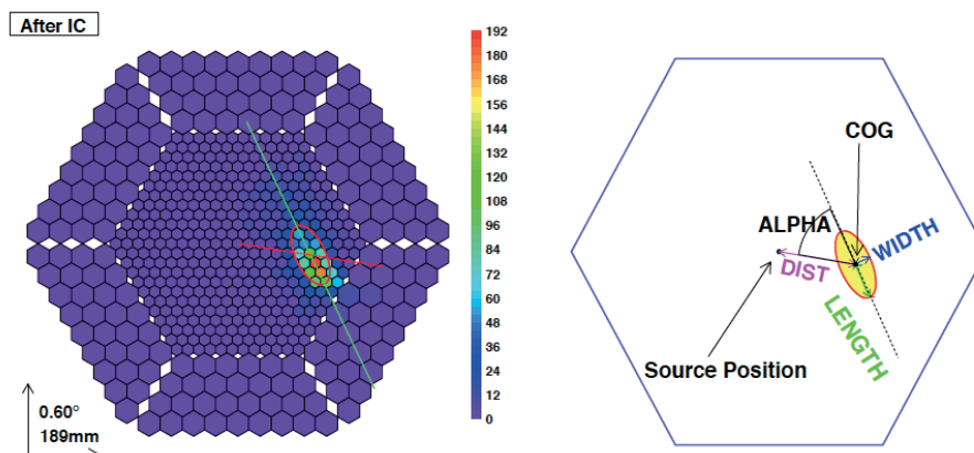
Abbildung 3.7: Beispielhafte Darstellung eines bereinigten Bildes und einiger Bildparameter in der alten MAGIC-Kamera.[43]
