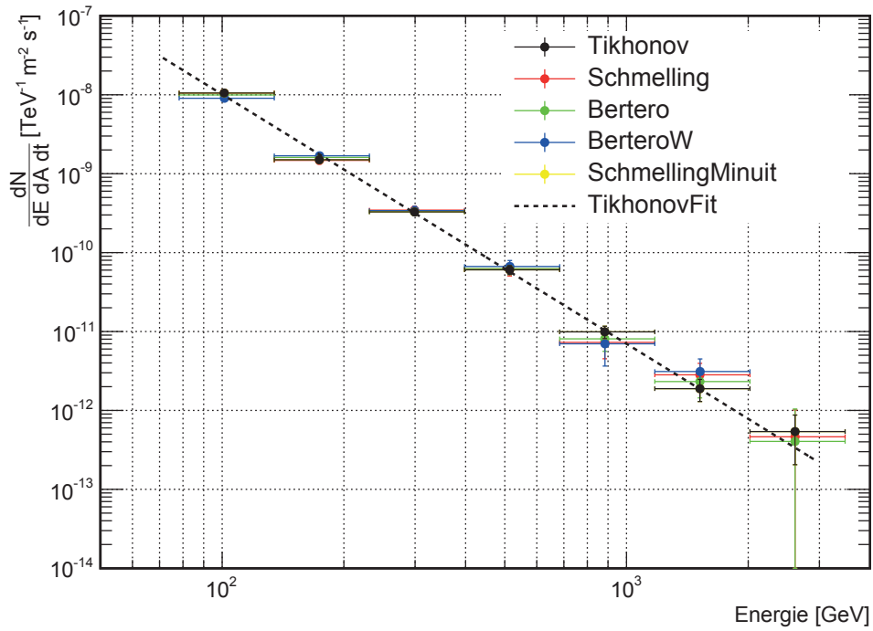
Abbildung 4.17: Entfaltetes Spektrum von Mrk 421 im Zeitraum vom 15.12.2012 bis zum 23.12.2012 mit allen wählbaren Regularisierungsmethoden. Die gestrichelte Linie stellt das gefittete Spektrum dar, welches mit Hilfe der Tikhonov-Regularisierung berechnet wurde.
