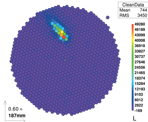
Abbildung 3.6: Darstellung des bereinigten Ereignisses in der Kamera.
