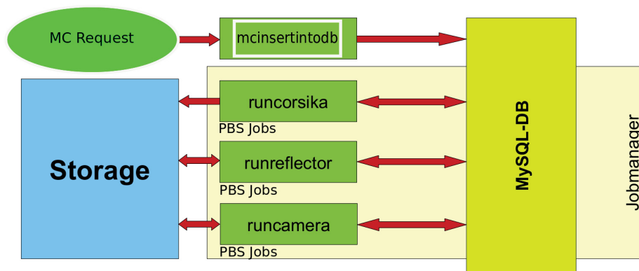
Abbildung 3.9: Schematische Darstellung der automatischen MC Produktionskette.
