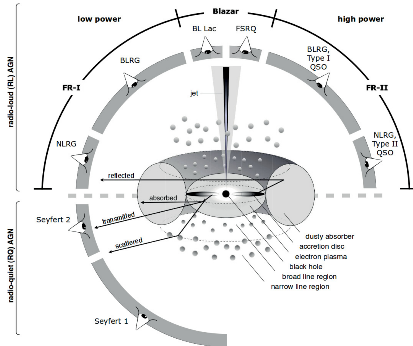
Abbildung 2.3: Schema zur Klassifikation von AGN (siehe Unterabschnitt 2.5.1). Abhängig von der Radioemission und dem Blickwinkel werden die einzelnen AGN-Typen voneinander unterschieden. Im Inneren einer AGN befindet sich ein supermassives Schwarzes Loch, welches von einer Akkretionsscheibe umgeben ist. Diese wird wiederum von einem Staubtorus umschlossen. Aus dem Zentrum werden zwei entgegengesetzte Jets emittiert.[14]
