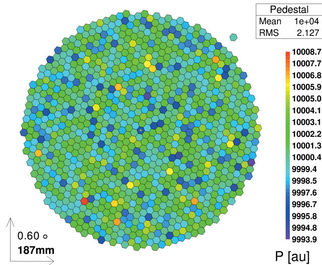
Abbildung 3.4: Darstellung eines simulierten Pedestal-Ereignisses in der Kamera. Dargestellt ist der Pixelinhalt in beliebigen Einheiten.
