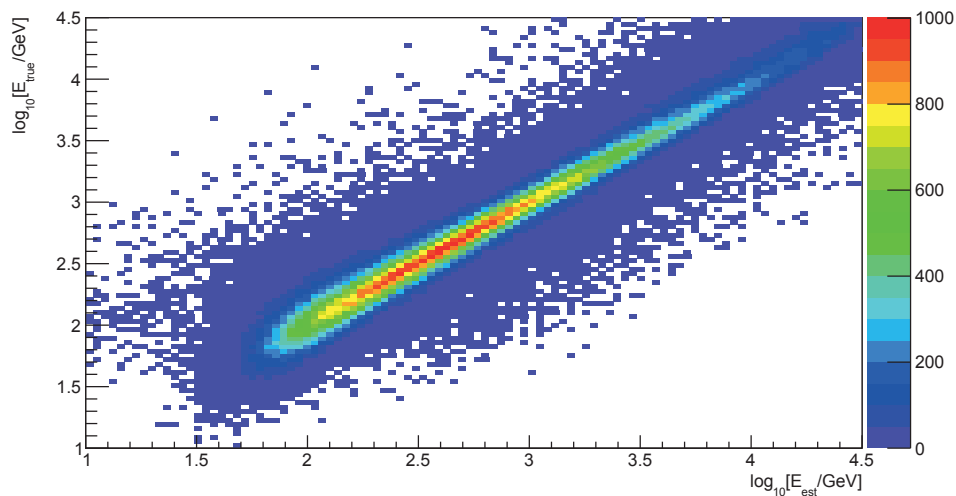
Abbildung 4.3: Dargestellt ist ein zweidimensionales Histogramm, in dem die geschätzte Energie gegen die wahre Energie aufgetragen ist. Es ist erkennbar, dass keine perfekte Energierekonstruktion existiert.
