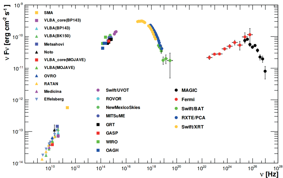
Abbildung 2.4: Die Abbildung zeigt die spektrale Energieverteilung von Mrk 421. Die für Blazare typische doppelhöckerige Struktur ist erkennbar. Des Weiteren ist zu sehen, dass das Maximum des niederenergetischen und des hochenergetischen Höckers einen ähnlichen Fluss aufweist.[2]
