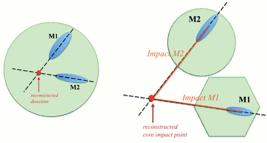
Abbildung 3.8: Rekonstruierte Richtung und rekonstruierter Core Impact-Punkt. Mit Hilfe der beiden Schauerbilder können sowohl die Herkunftsrichtung des Schauers, als auch der Punkt, in dem die Schauerachse den Boden trifft rekonstruiert werden.[45]
