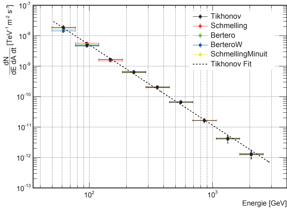
Abbildung 4.11: Entfaltetes Mrk 421-Spektrum im Zeitraum vom 18.3.2012 bis zum 25.4.2012 mit allen wählbaren Regularisierungsmethoden. Die gestrichelte Linie stellt das gefittete Spektrum dar, welches mit Hilfe der Tikhonov-Regularisierung berechnet wurde.
